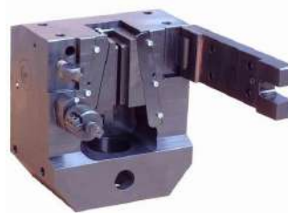
300 kN Wedge Action Grip
